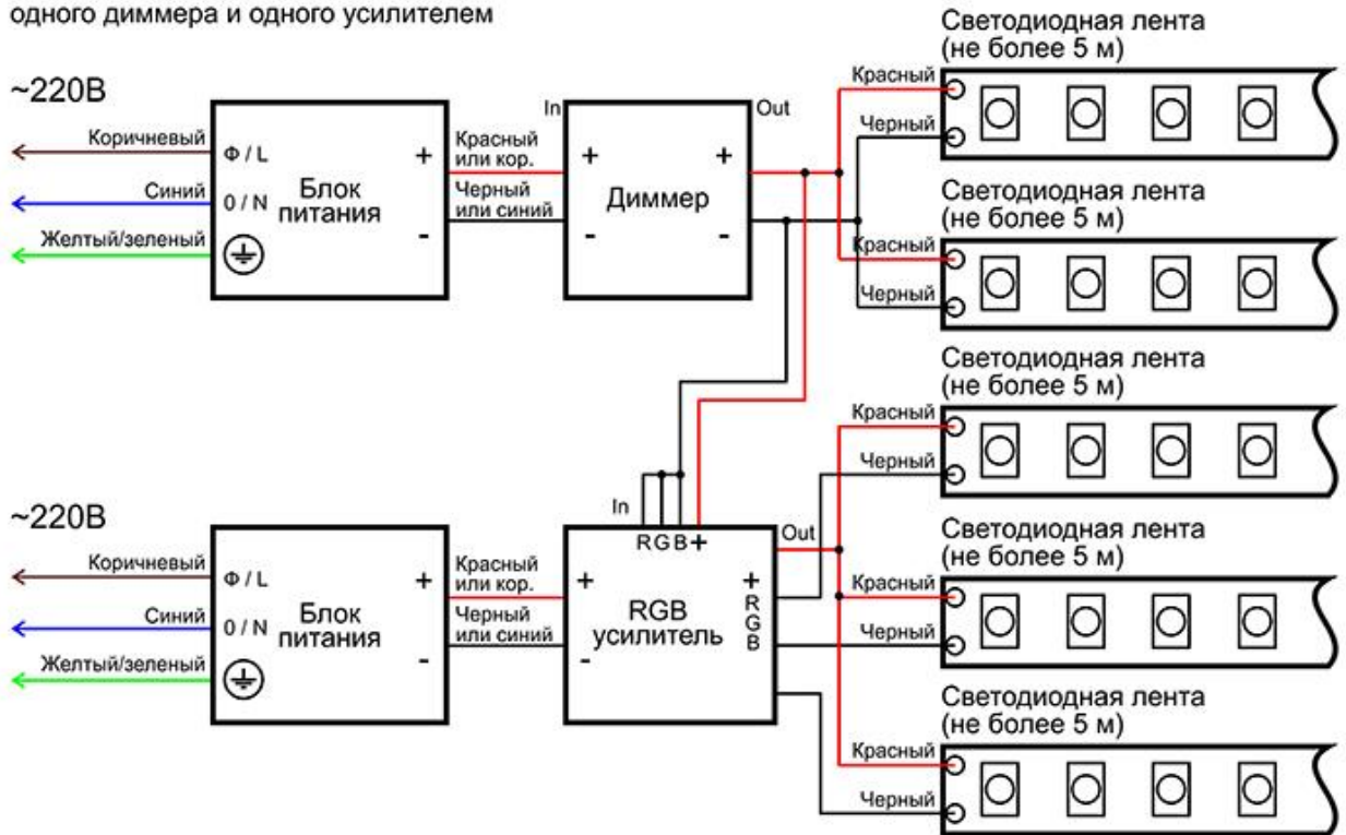
Схема подключения монохромной ленты с использованием одного диммера и одного усилителем
