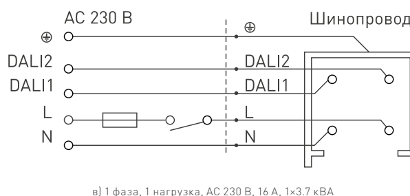
Рисунок 3. Схема подключения
