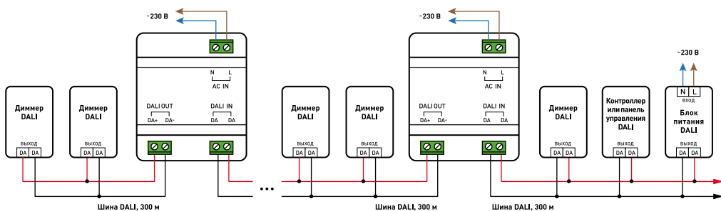
Рис. 2. Схема подключения DALI-302-REP-DIN в качестве усилителя-ретранслятора сигнала DALI
